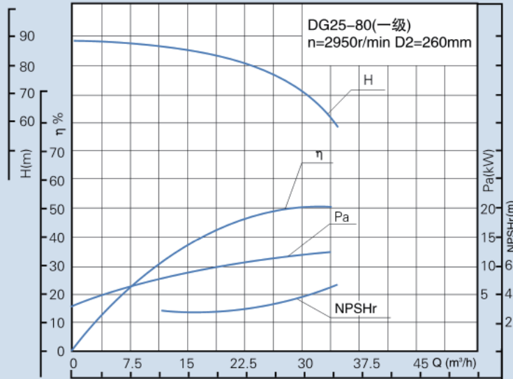
CMB25-80次高压泵性能表
