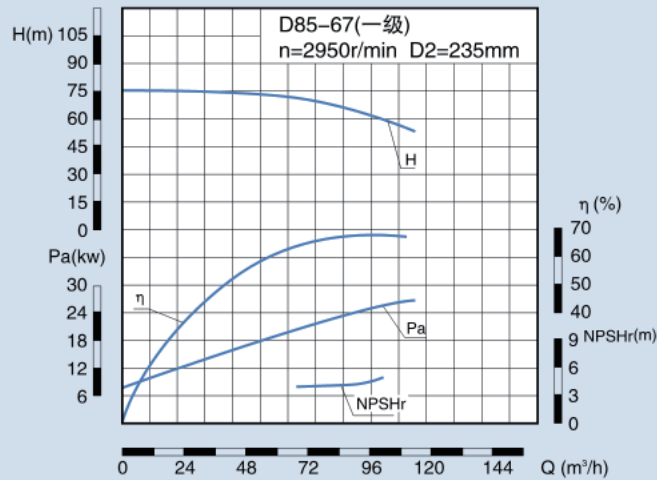
CMB 85-67 性能表
