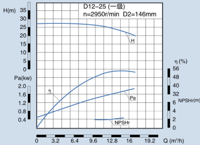
CMB 12-25 性能表
