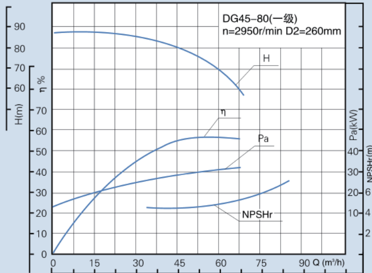
CMB 45-80次高压泵性能表
