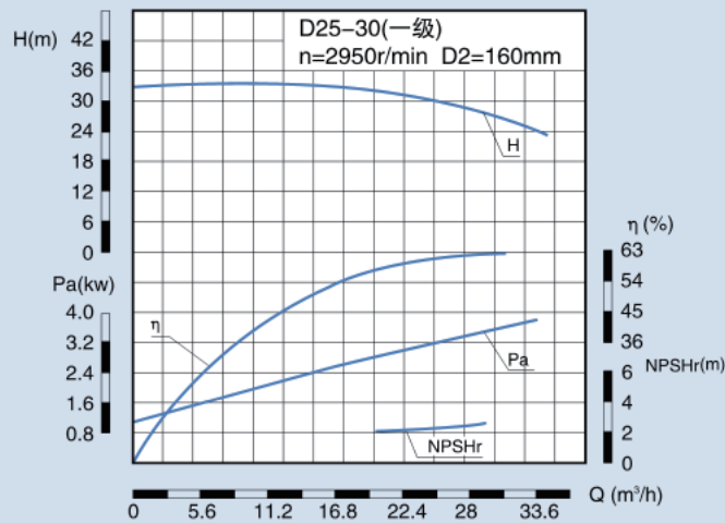
CMB 25-30 性能表
