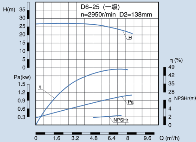
CMB 性能表
