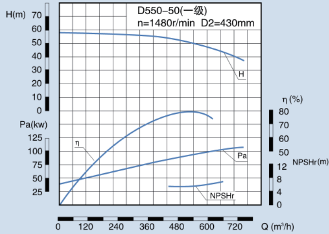
CMB 550-50 性能表
