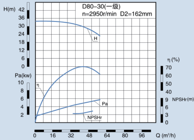
CMB 80-30 性能表
