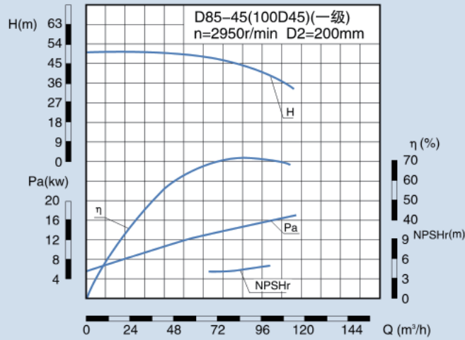
CMB 85-45(100 45) 性能参数表
