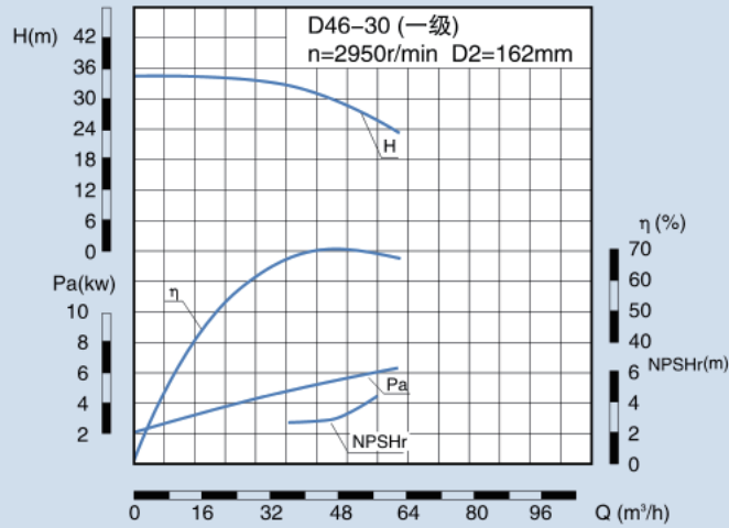
CMB 46-30 性能表
