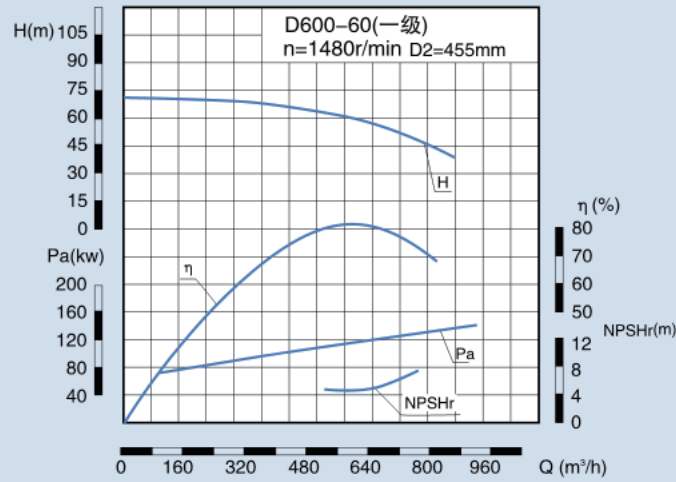
CMB600-60性能表
