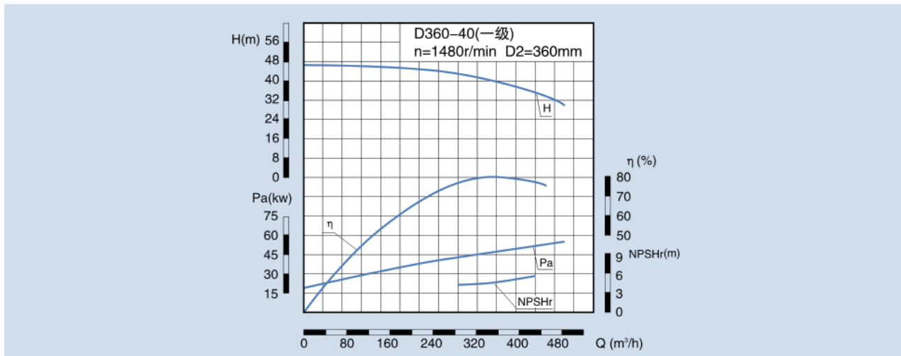
CMB 360-40 性能表
