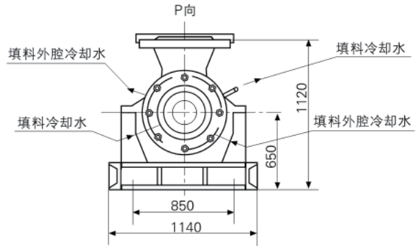
CMB 150-100次高压泵外形安装尺寸表 CMB150-100 Installation Dimensions
