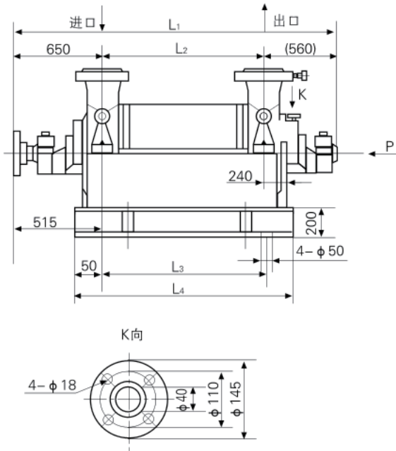
CMB 150-100型次高压泵外形安装图
