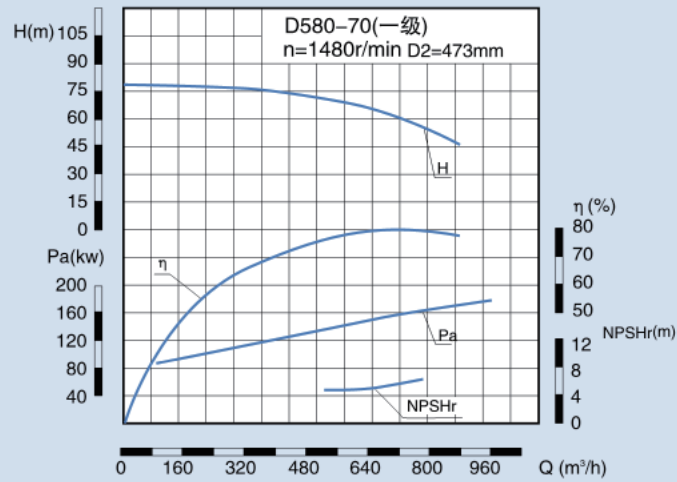
CMB580-70性能表
