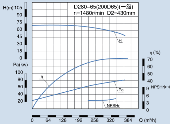
CMB 280-65(200 65) 性能表
