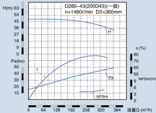
CMB 280-43(200 43) 性能表
